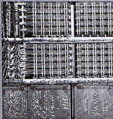
Particolare del telaio « accoppiatori » della nuova centrale semielettronica, attivata a Roma-EUR, che utilizza relé elettromagnetici ESK.
