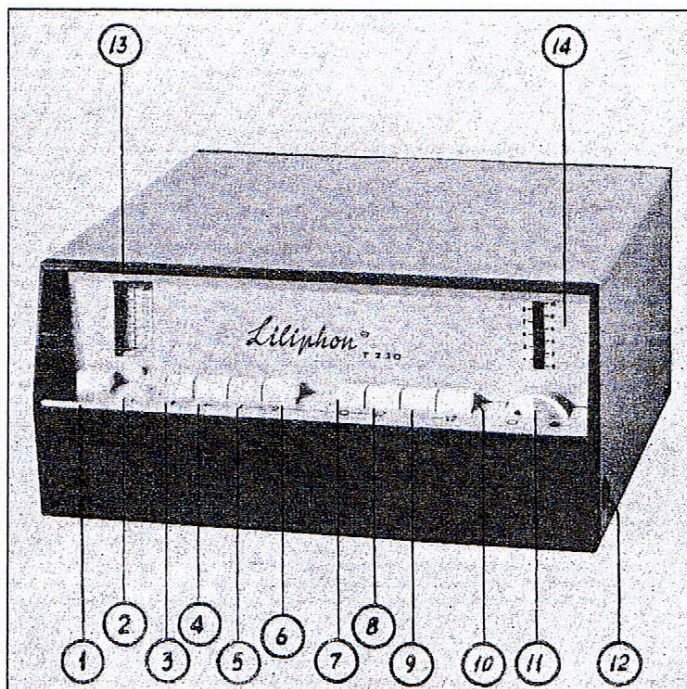
Segretario telefonico automatico del tipo « Liliphon T 230 » della Casa Gnechchi di Milano. Può trasmettere due annunci e registrare fino a 30 messaggi in arrivo, di 30, 45 e 60 secondi ciascuno. Descrizione: 1: tasto per la cancellazione totale; 2: pulsante di azzeramento della scala; 3: tasto per far salire l'indice della scala; 4: tasto di avviamento manuale; 5: tasto per « 1° Teste Annuncio »; 6: tasto per « 2° Annuncio »; 7: tasto per la registrazione dei testi annunci; 8: tasto per l'ascolto dei testi annunci; 9: tasto per il funzionamento telefonico automatico; 10: tasto per l'ascolto dei messaggi ricevuti; 11: interruttore e regolatore del volume di ascolto; 12: presa per microfono; 13: scala per la scelta dei messaggi; 14: scala di controllo del tempo di registrazione annunci.
